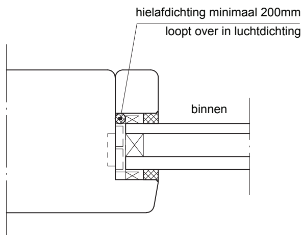
stijlen kozijnen, ramen, deuren en (hef)schuifdeuren
