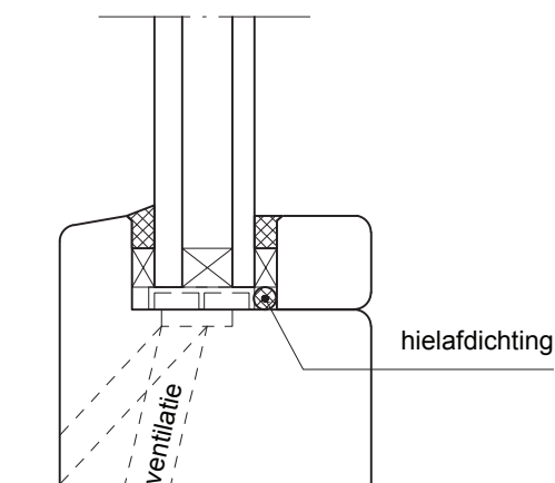
binnenbeglazing onderdorpel ramen, deuren, (hef)schuifdeuren
